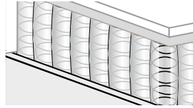
Tonnen-Taschenfederkern 1000 Federn
