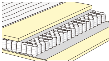
Taschenfederkern mit 500 Federn
